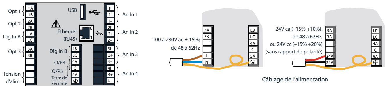
Borniers arrières
