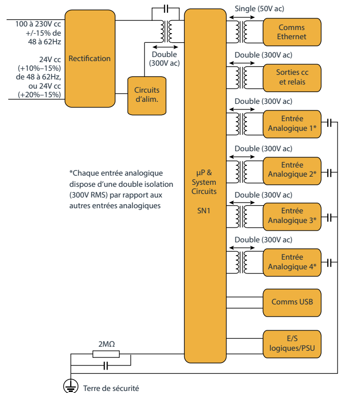
Détails d'isolation
