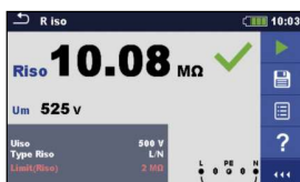
Mesure d'isolement
