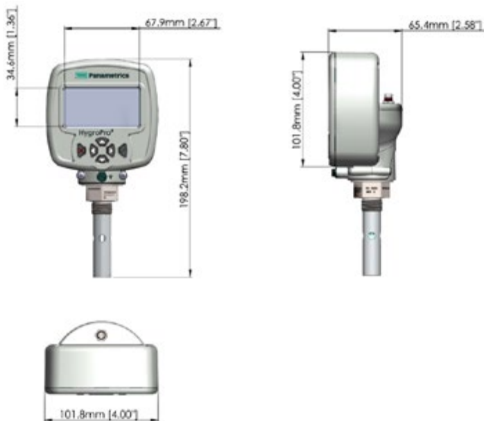
HygroPro ® dimensions
