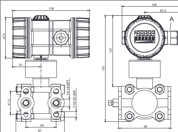
Type 403022/0-0-2 (long, acier inoxydable avec presse-étoupe)
