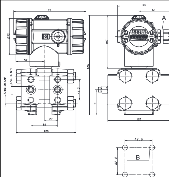
avec option 694 (pression nominale augmentée PN420)
