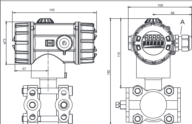
Type 403022/0-0-3 (moulage de précision avec presse-étoupe)
