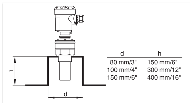
Fig. 8: Autres dimensions de rehausse
