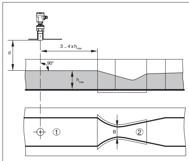
Fig. 16: Mesure de débit avec canal Venturi Khafagi : d = distance de blocage du capteur ; h_{max} = remplissage max. du canal ; B = étranglement maximum du canal
