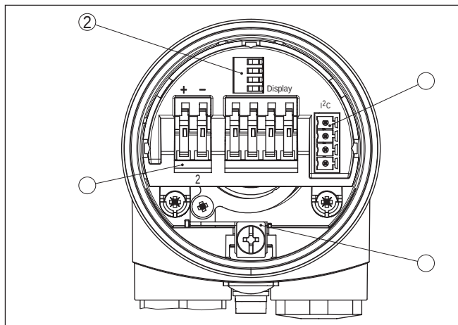
Fig. 19: Compartiment électronique et de raccordement de boîtier à chambre unique
