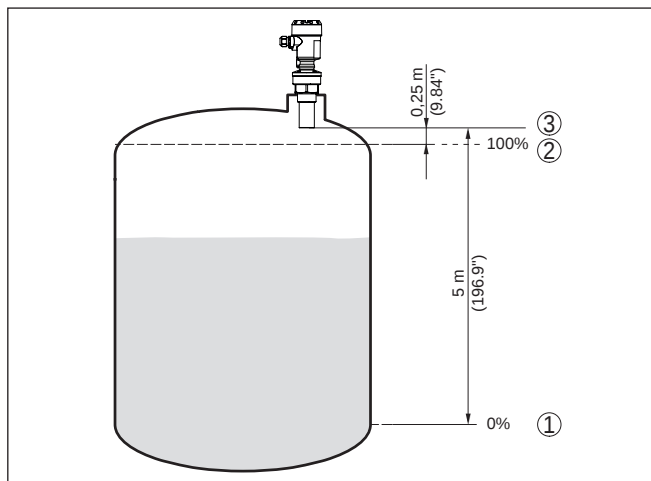
Fig. 27: Exemple de paramétrage réglage min./max.
