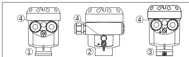
Fig. 18: Boîtier à chambre unique proposé en plusieurs matériaux
