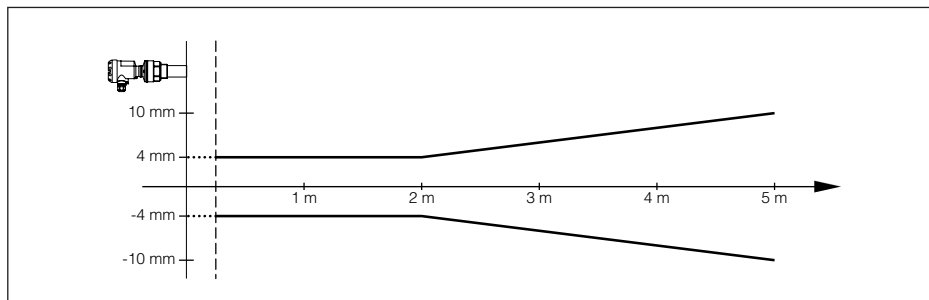
Fig. 29: Écart de mesure OPTISOUND 3010 C
