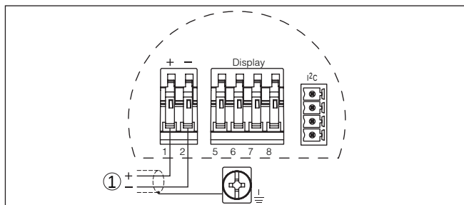
Fig. 20: Schéma de raccordement - boîtier à chambre unique
