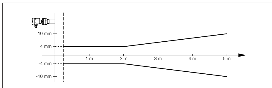
Fig. 28: Écart de mesure OPTISOUND 3010 C
