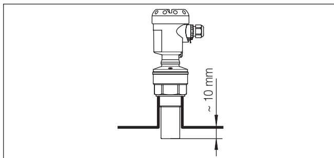
Fig. 7: Montage sur rehausse recommandé
