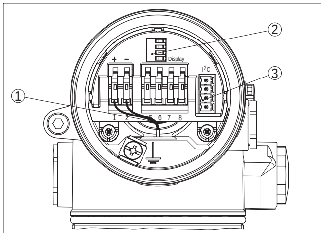
Fig. 22: Compartiment électronique - boîtier à deux chambres
