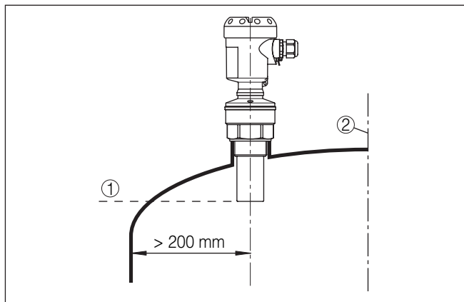
Fig. 5: Montage sur cuve à toit bombé
