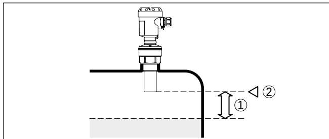
Fig. 3: Distance de blocage jusqu'à la hauteur de remplissage max.
