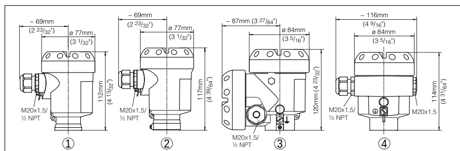
Fig. 30: Variantes de boîtier en protection IP66/IP67 et IP66/IP68 ; 0,2 bar (avec un module de réglage et d'affichage intégré, la hauteur du boîtier augmente de 9 mm/0.35 in pour les boîtiers en plastique, et de 18 mm/0.71 in pour les boîtiers métalliques)
