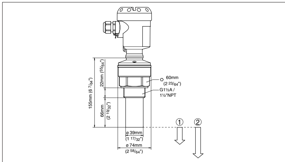
Fig. 31: OPTISOUND 3010 C
