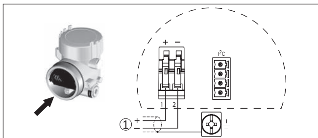
Fig. 24: Schéma de raccordement - boîtier à deux chambres
