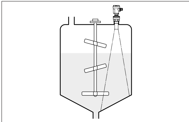
Fig. 12: Agitateurs
