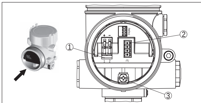
Fig. 23: Compartiment de raccordement boîtier à deux chambres
