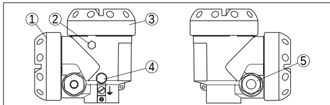
Fig. 21: Boîtier à deux chambres
