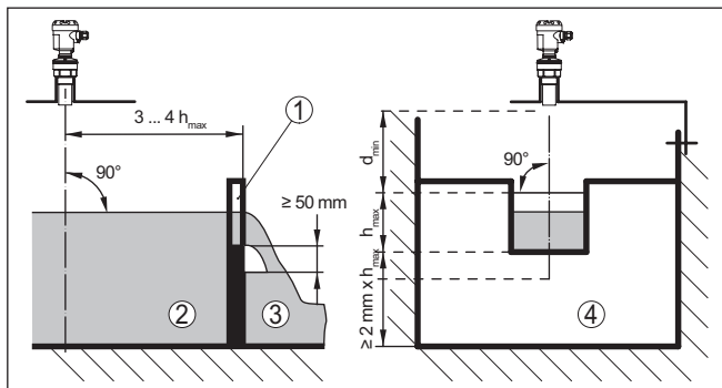
Fig. 15: Mesure de débit avec déversoir rectangulaire : d_{\min} = distance de blocage du capteur (voir chapitre "Caractéristiques techniques") ; h_{\max} = remplissage max. du déversoir rectangulaire
