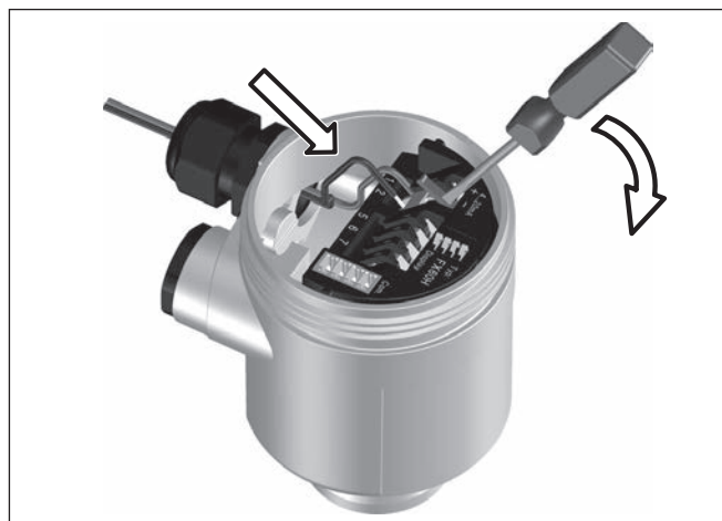
Fig. 17: Étapes de raccordement 6 et 7
