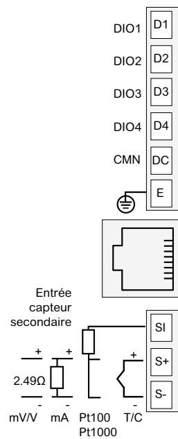
ENTRÉE PV ETHERNET 4 x ENTRÉES / SORTIES LOGIQUES
