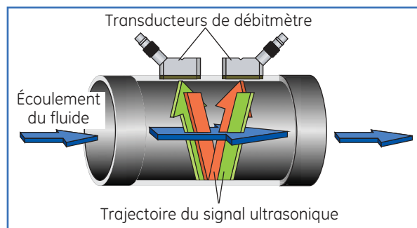
Technique de mesure du débit à temps de transit
